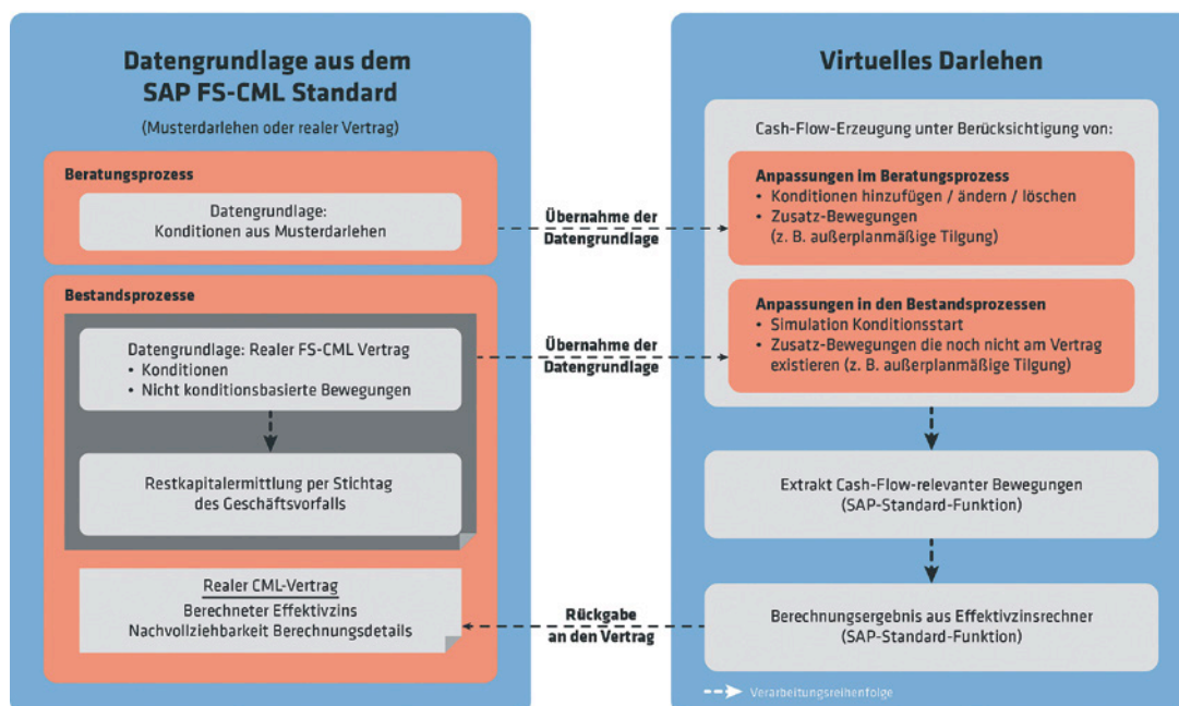
Virtuelles Darlehen als Lösung für die Effektivzinsberechnung in SAP FS-CML
